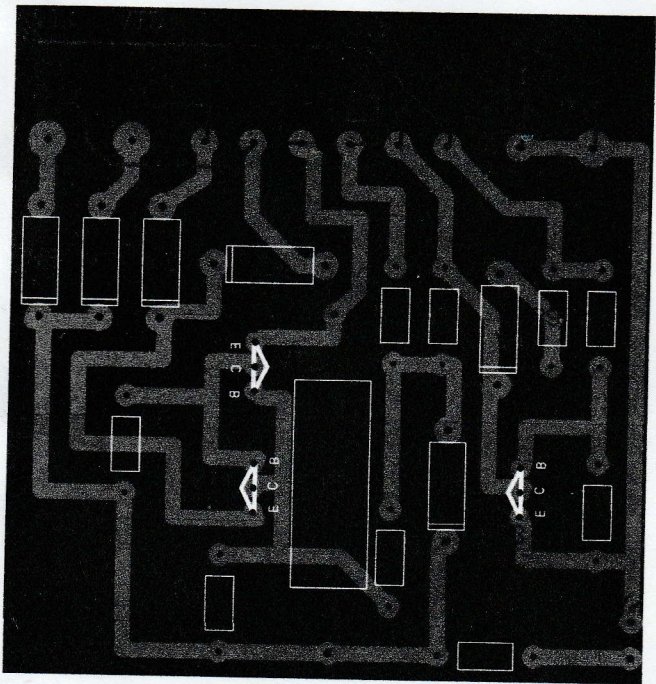
Рис.2. Печатная плата
